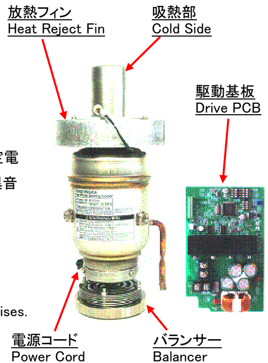
SC-TD08 スターリングクーラー 08 SC-TD08 Stirling Cooler 08
